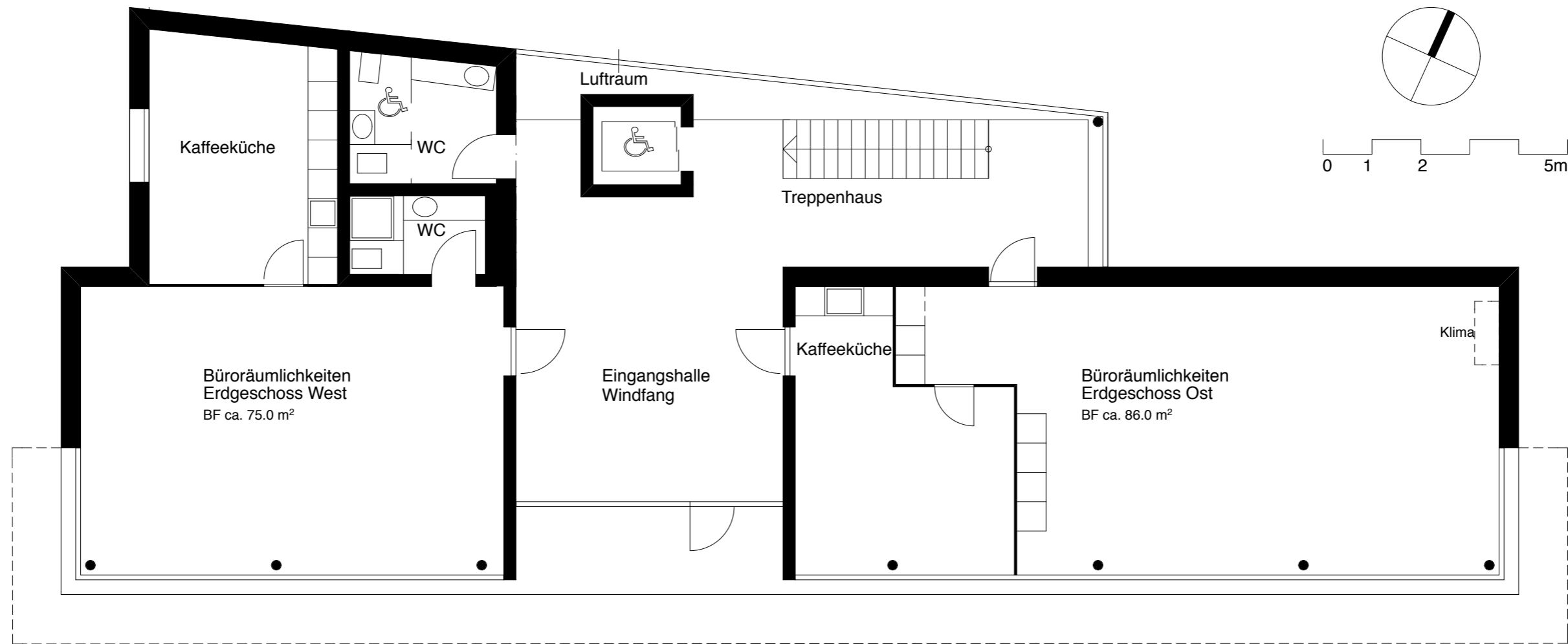
Grundriss Erdgeschoss
